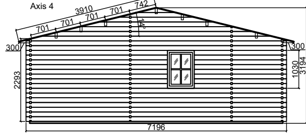
Axis 4
